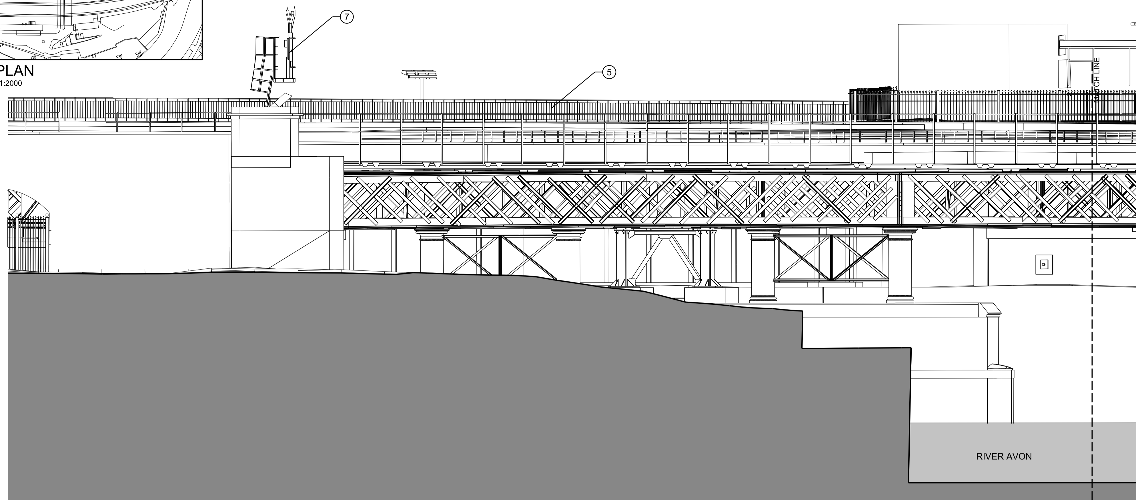
ELEVATION 1
